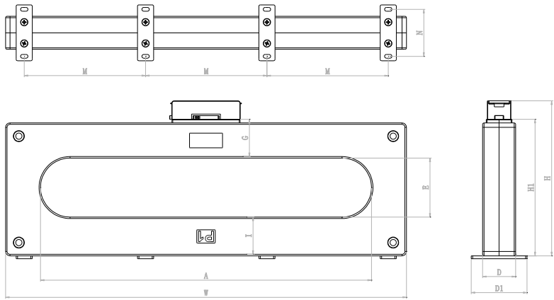
图 5 探测器外形示意图（配闭 DH-GST-N2200-F-2000 剩余电流互感器）
