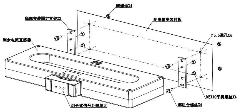
图10 探测器安装过程分解图（配 DH-GST-N2200-F-1000 剩余互感器）
