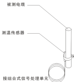
图 13 测温传感器安装图
