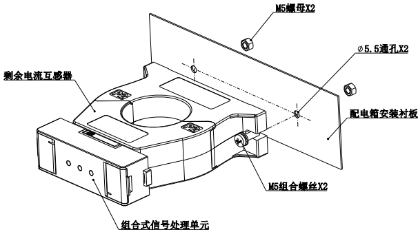
图 12 探测器安装过程分解图（配圆形开口式剩余电流互感器）
