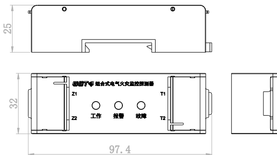
图 1 探测器信号处理单元外形示意图
