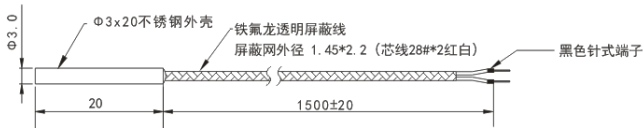
图 7 测温传感器结构尺寸图
