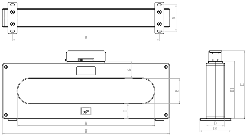
图 4 探测器外形示意图（配闭 DH-GST-N2200-F-1000 剩余电流互感器）
