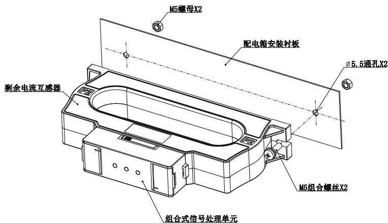
图9 探测器安装过程分解图（配方形剩余电流互感器）
