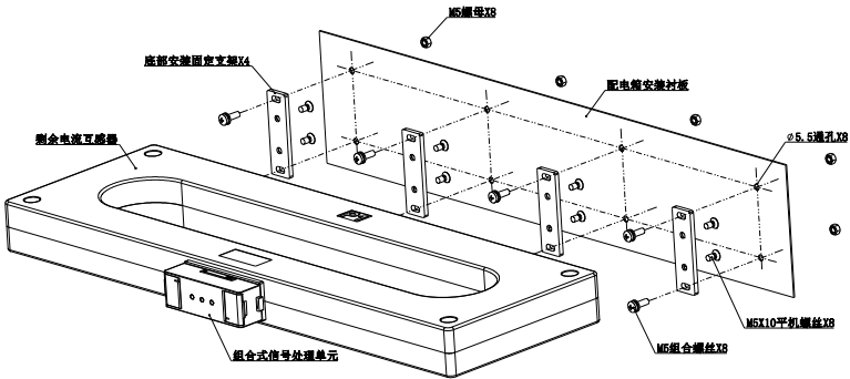
图 11 探测器安装过程分解图（配 DH-GST-N2200-F-2000 剩余互感器）
