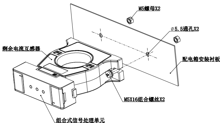
图 8 探测器安装过程分解图（配闭口式圆孔剩余电流互感器）
