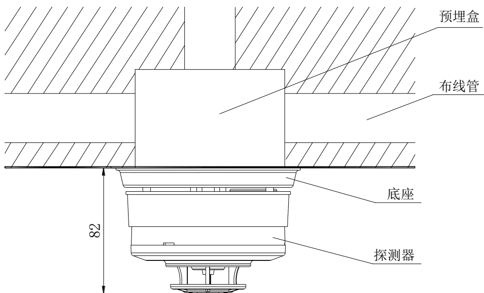
图 2 探测器安装示意图
