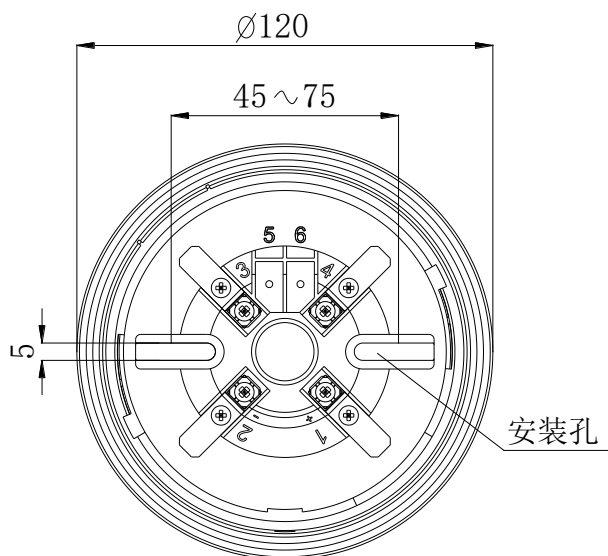
图3 底座外形示意图
