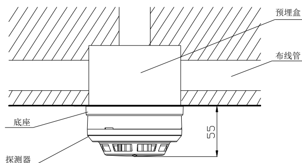
图 2 探测器安装示意图
