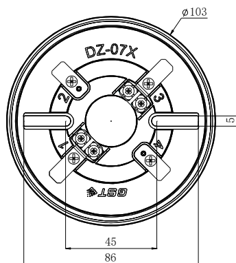
图3 探测器底座(DZ-07X)外形示意图
