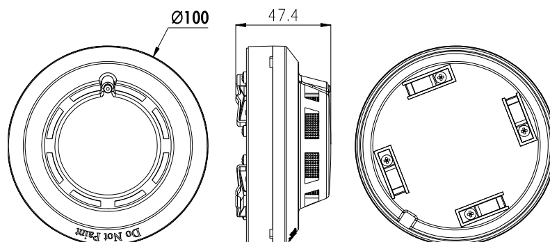
图 1 探测器外形示意图
