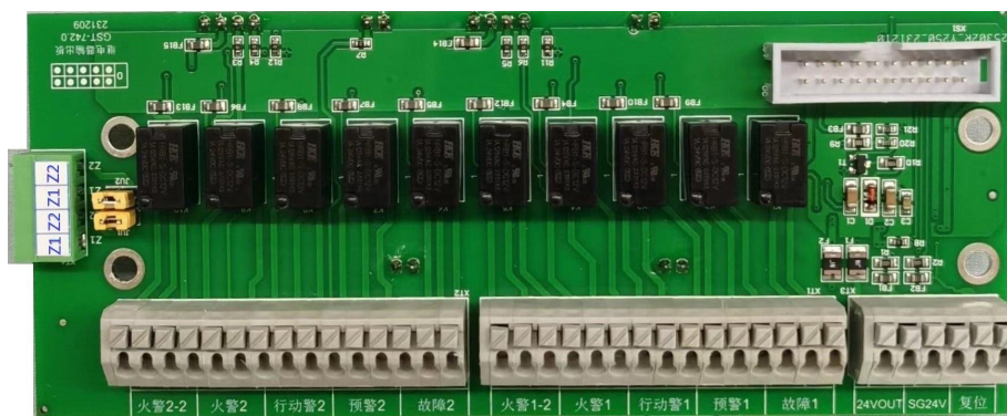
图 4.3 继电器板与外部连接示意
