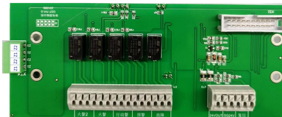
图 4.3 继电器板与外部连接示意
