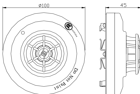
图 1 探测器外形示意图
