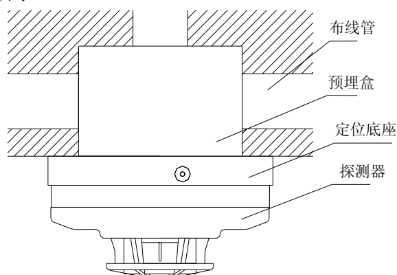
图 2 探测器安装示意图
