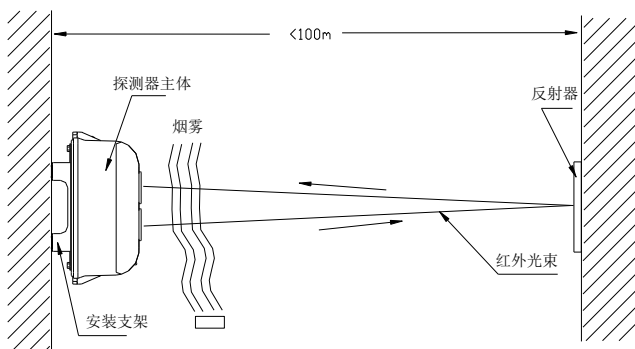
图 3 工作原理图
