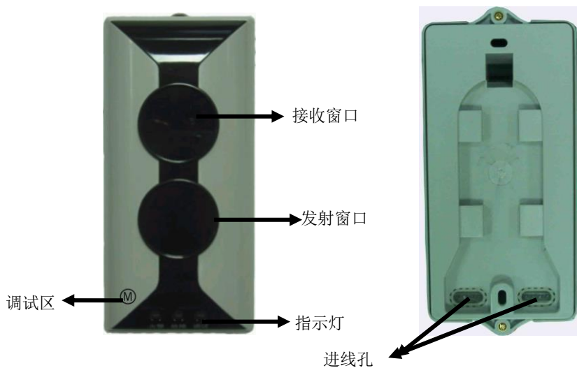
图 1 探测器外形示意图
