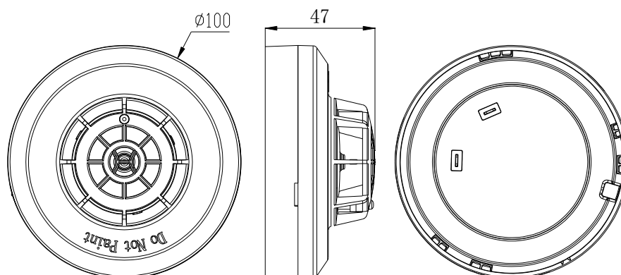
图 1 探测器外形示意图
