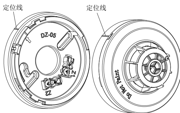
图 4 探测器与底座安装示意图
