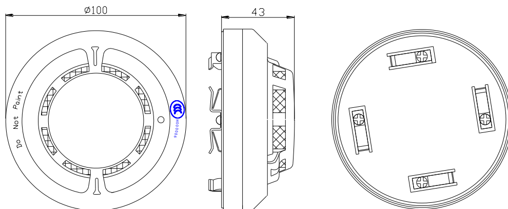
图1 探测器外形示意图
