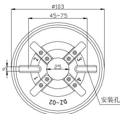
图3 探测器通用底座外形示意图
