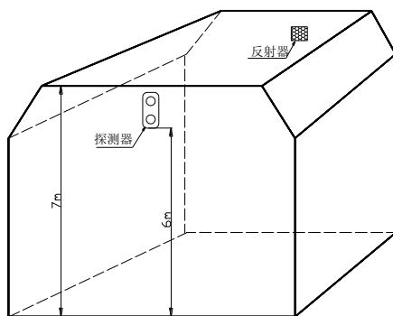
图 5 探测器和反射器安装示意图
