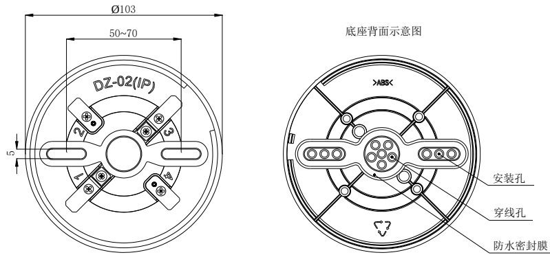
图 3 探测器 DZ-02(IP)底座外形示意图
