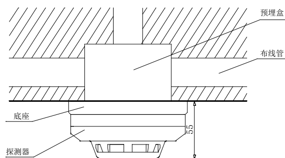
图 2 探测器安装示意图
