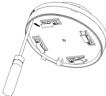
图 5 敲落泄水孔示意图
