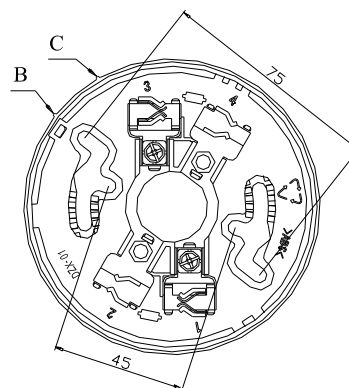
图4 DZX-01 定位底座外形示意图
