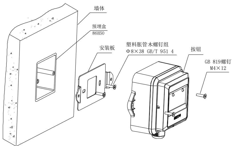
图 3 安装示意图
