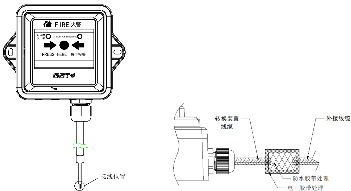
图 5 接线示意图
