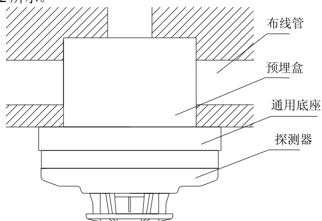
图2 探测器安装示意图
