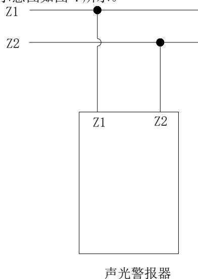
图 4 警报器信号总线接线示意图
