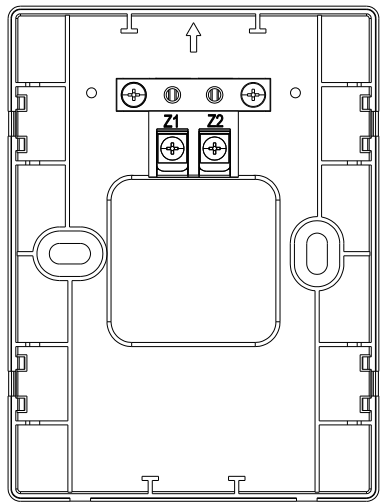
图 3 底壳示意图
