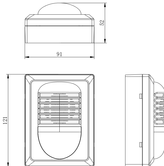
图 1 警报器外形示意图
