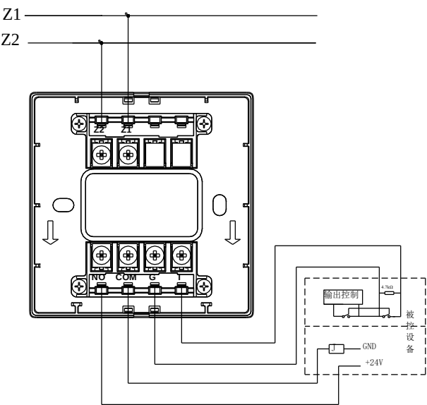
图 4 输入常开检线示意图
