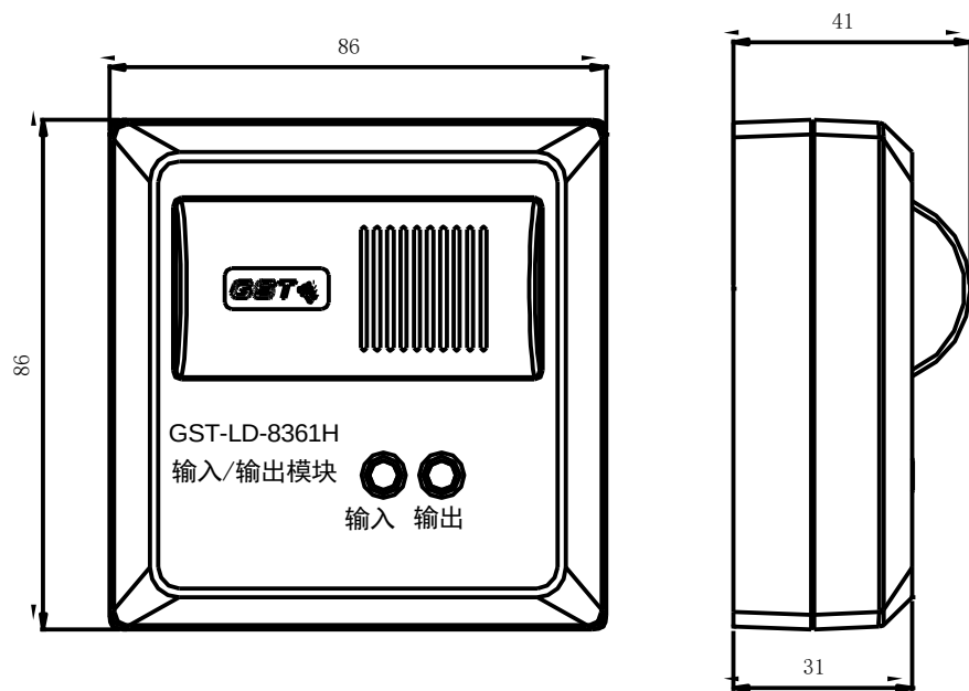
图1 外形示意图
