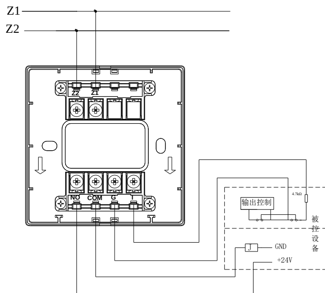
图 5 输入常闭检线示意图
