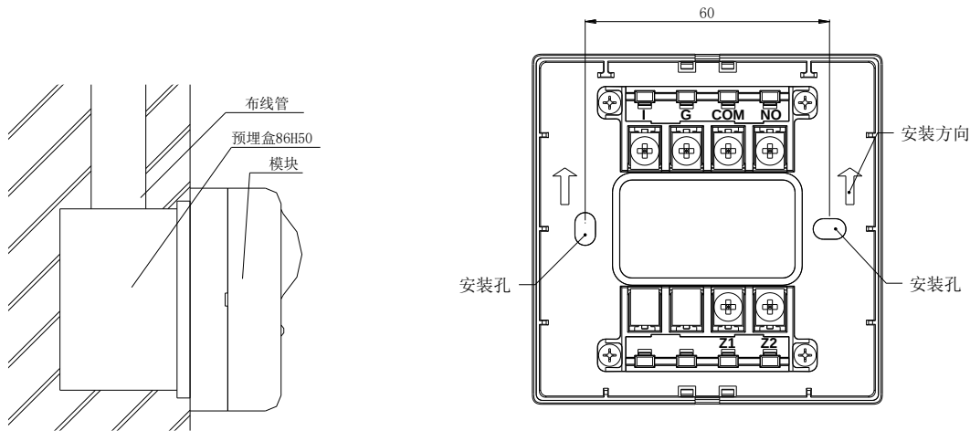
图2 进线管预埋示意图
