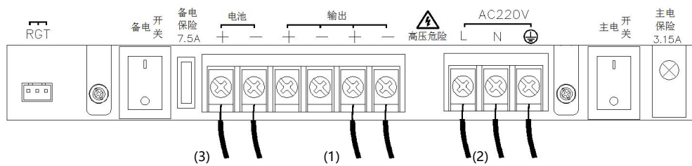
图 2 外接端子示意图
