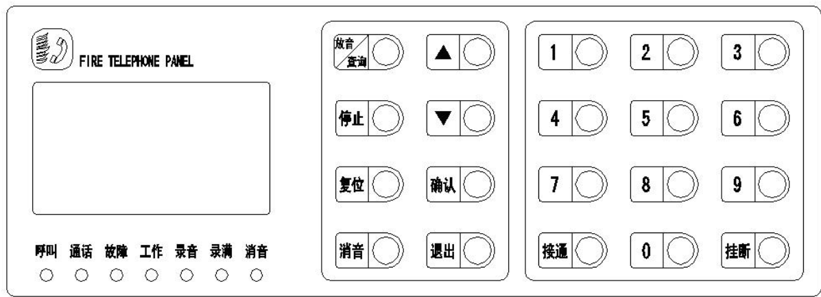
图 4.2 TSZ-GSTN60 消防电话总机操作显示区示意图
