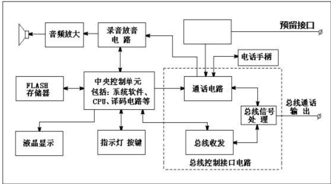
图 3.2 TSZ-GSTN60 消防电话总机原理结构框图
