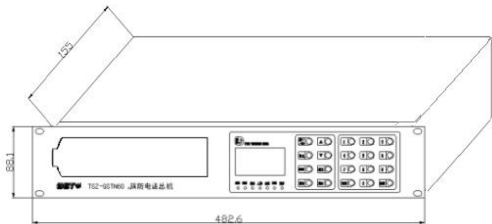
图 4.1 TSZ-GSTN60 消防电话总机外形示意图
