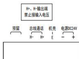
图 3.4 TSZ-GSTN60 消防电话总机后面板示意图
