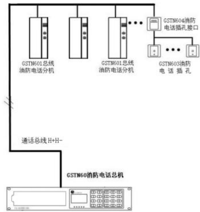
图 3.1 TS-GSTN60 消防电话系统构成图
