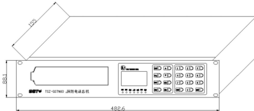
图 2 TS-GSTN60 消防电话总机外形示意图
