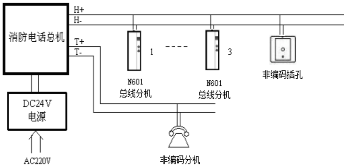
图 7 特殊应用示意图
