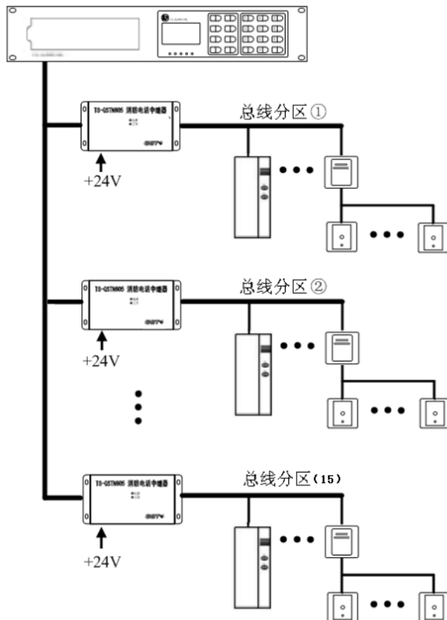
图 5 系统“总线分区”示意图
