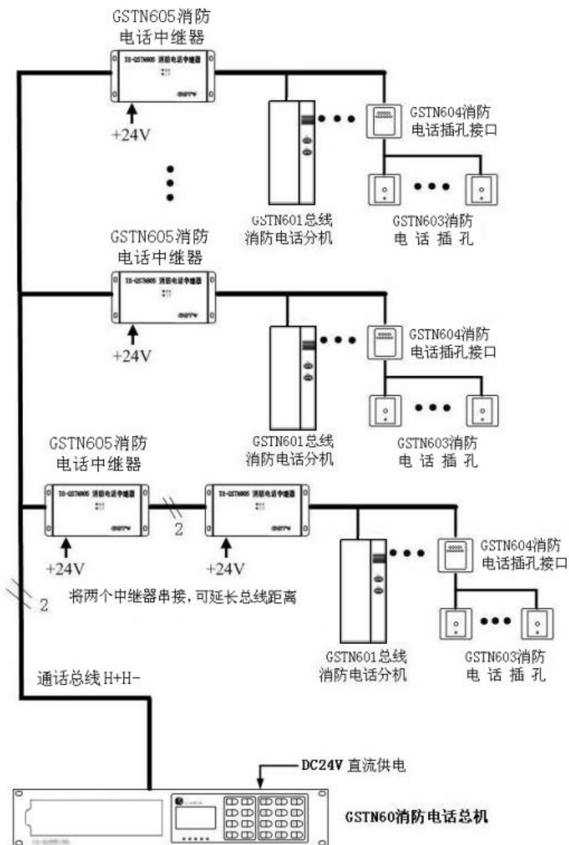
图 1 TS-GSTN60 两总线消防电话系统构成图
