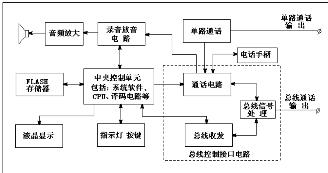
图 4 TS-GSTN60 消防电话总机原理结构框图
