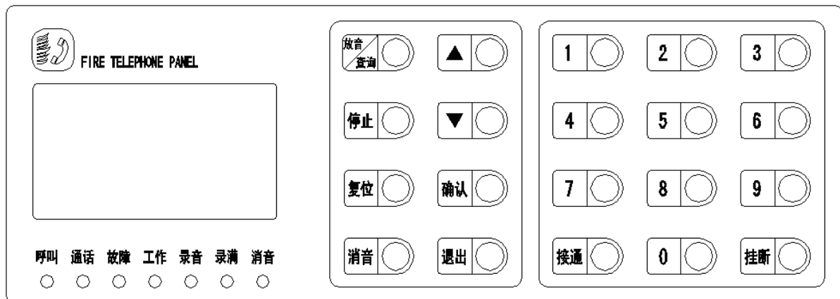
图 3 TS-GSTN60 消防电话总机操作显示区示意图
